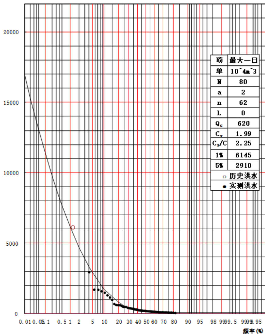
图3.2-5 福利屯站最大一日流量频率曲线图
